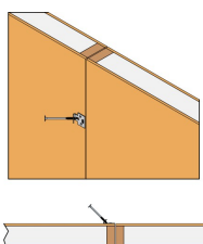
Mise en oeuvre entre panneaux bois: insérer la vis SDW
