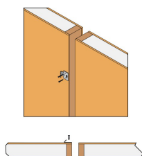
Mise en oeuvre entre panneaux bois: insérer les 2 pointes torsadées
